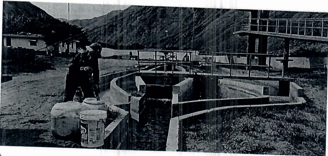
Captación Bocatoma "El Canuto"
