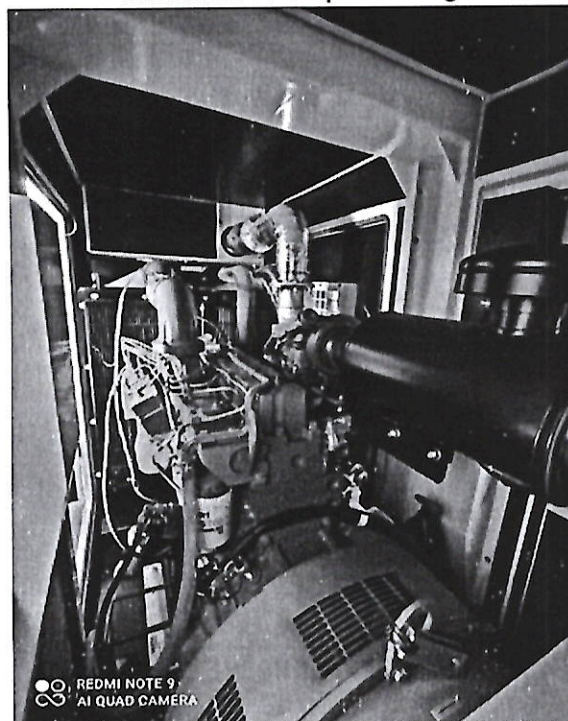
Ilustración 11 Grupo Electrónico
