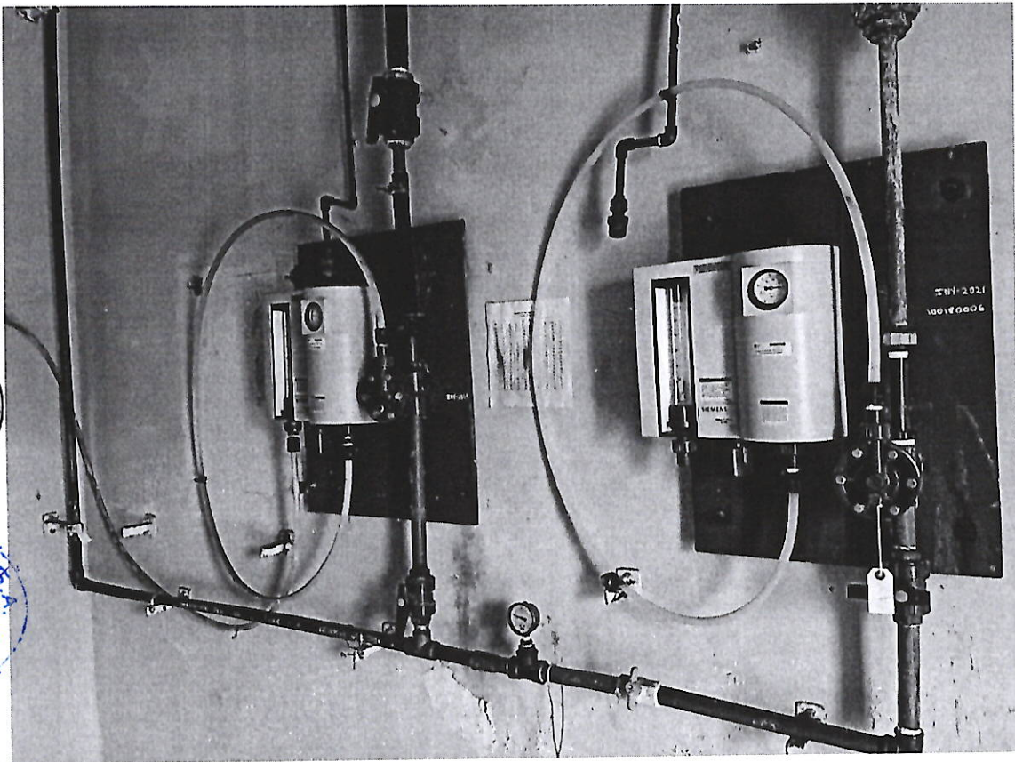
Ilustración 30 Clorinadores
