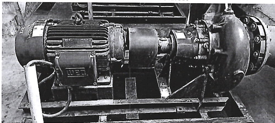
Ilustración 24 Bomba de lavado
