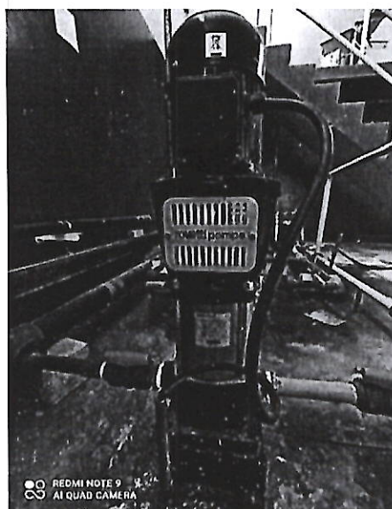
Ilustración 28 Electrobomba sobrepresión 2
