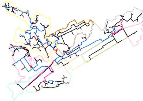
Líneas de agua potable (primarias)
