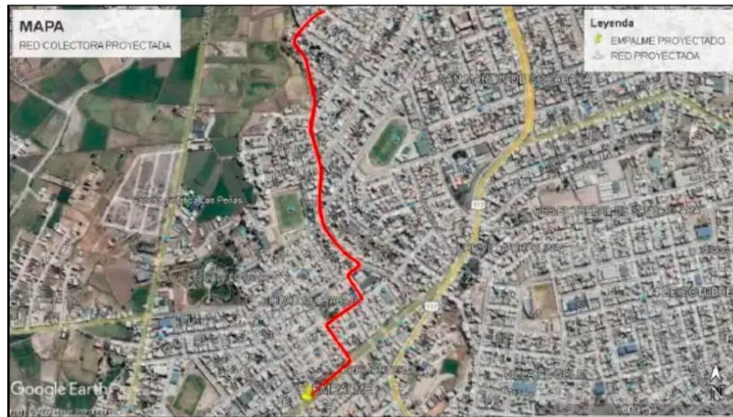
IMAGEN 9. PLANO DE INTERVENCIÓN EN SOCABAYA EJECUTADO POR SEDAPAR
