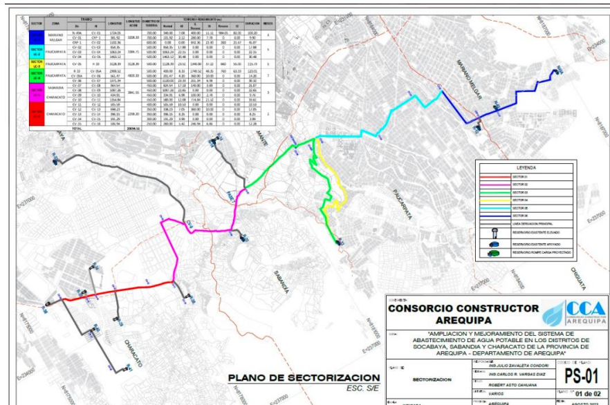
IMAGEN 8. PLANO DE SECTORIZACIÓN EN EL PROYECTO SOCABAYA, SABANDIA Y CHARACATO DE SEDAPAR
